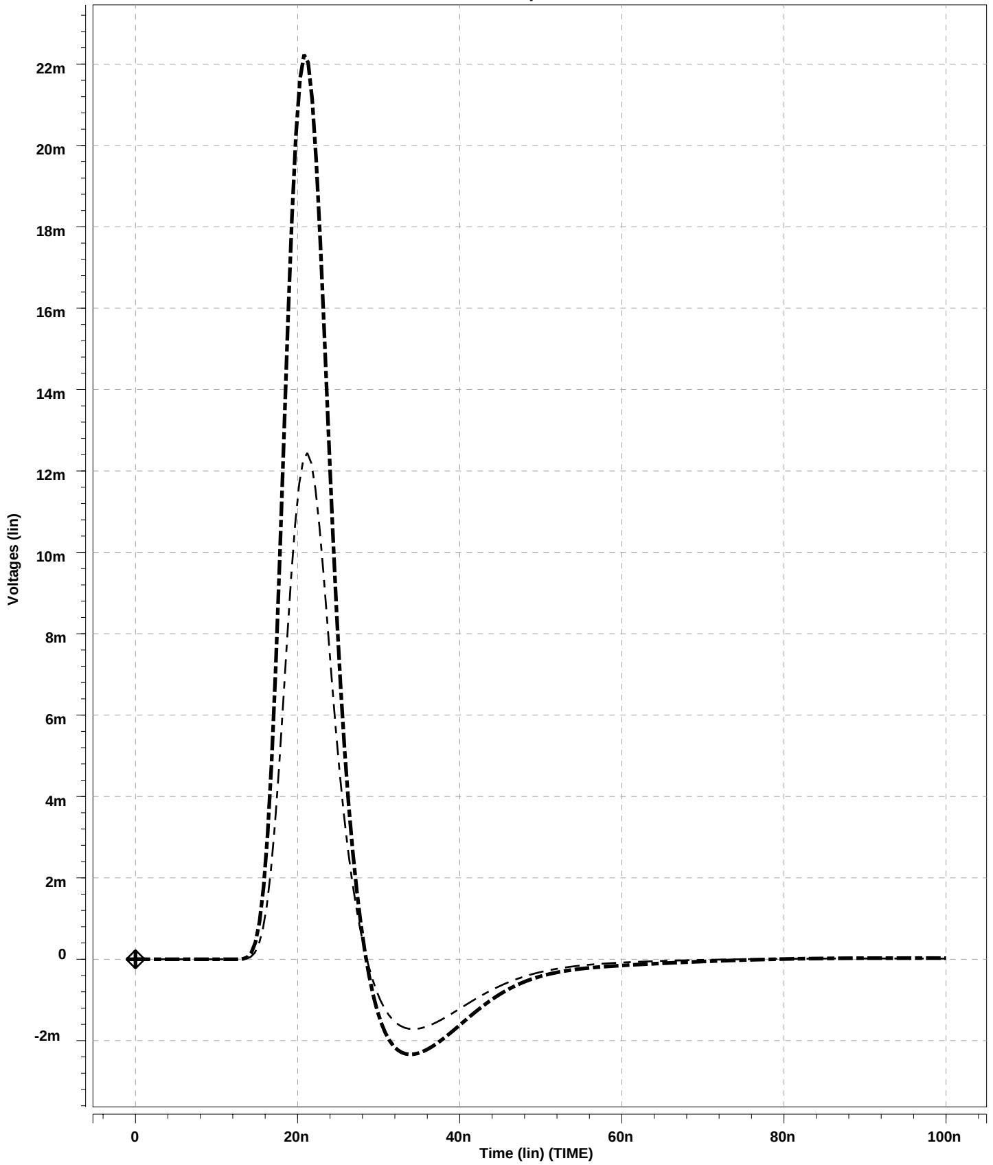
ASDBLR00 vs ASDBLR02 Track Disc Input Xe 100%e 2fC Beta=250
