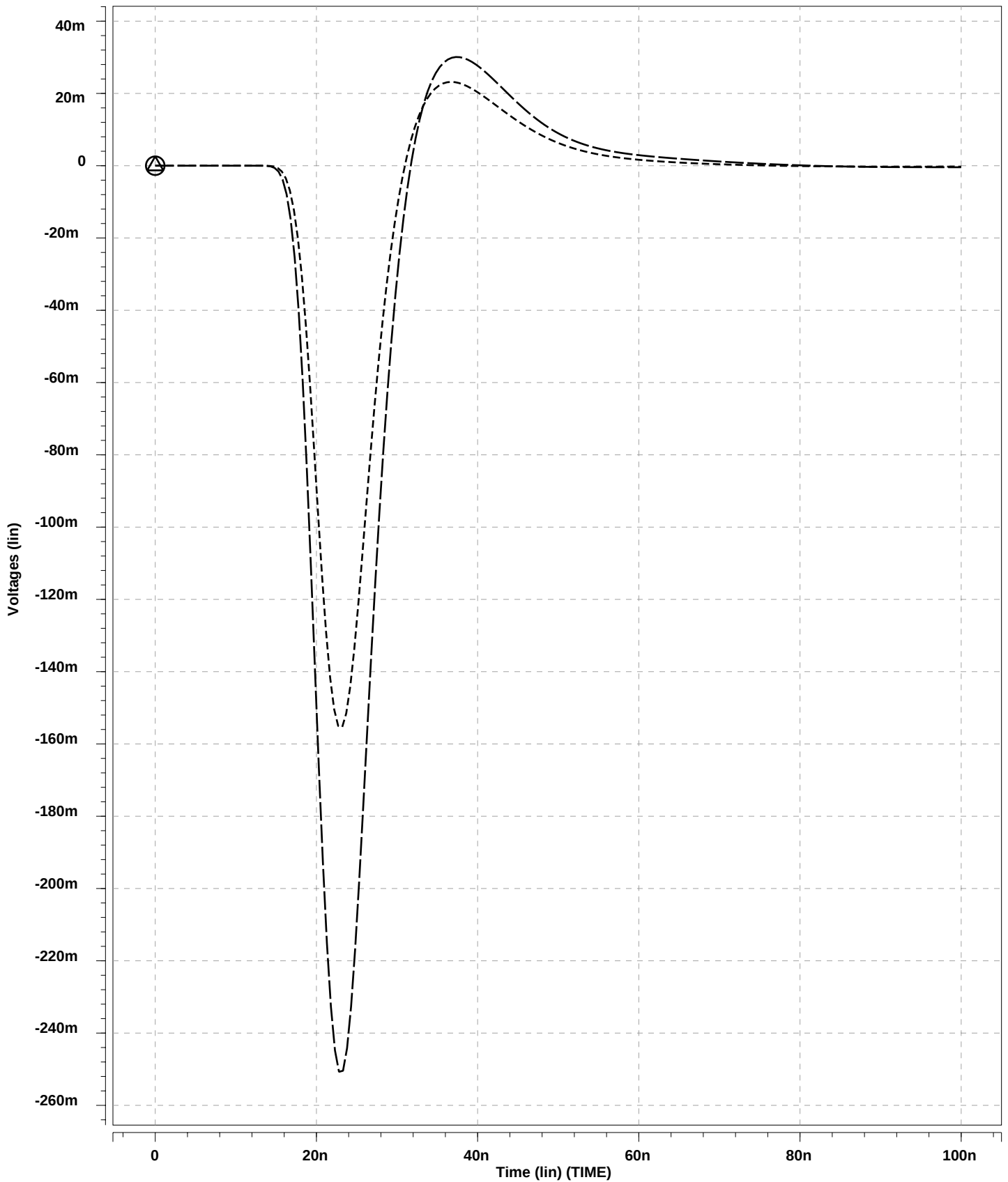
ASDBLR00 vs ASDBLR02 Track Disc Col Xe 100%e 2fC Beta=250
