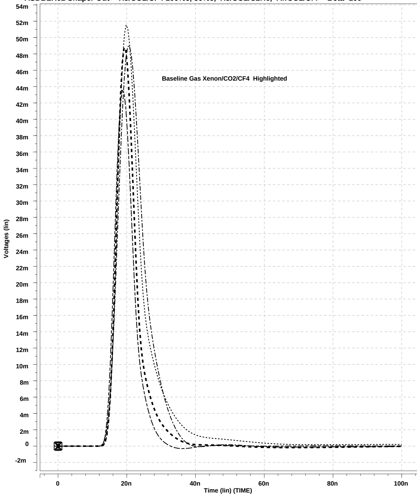
ASDBLR02 Shaper Out -- Xe/CO2/CF4 100%e, 50%e, Xe/CO2/C2H6, Ar/CO2/Cf4 -- Beta=100
