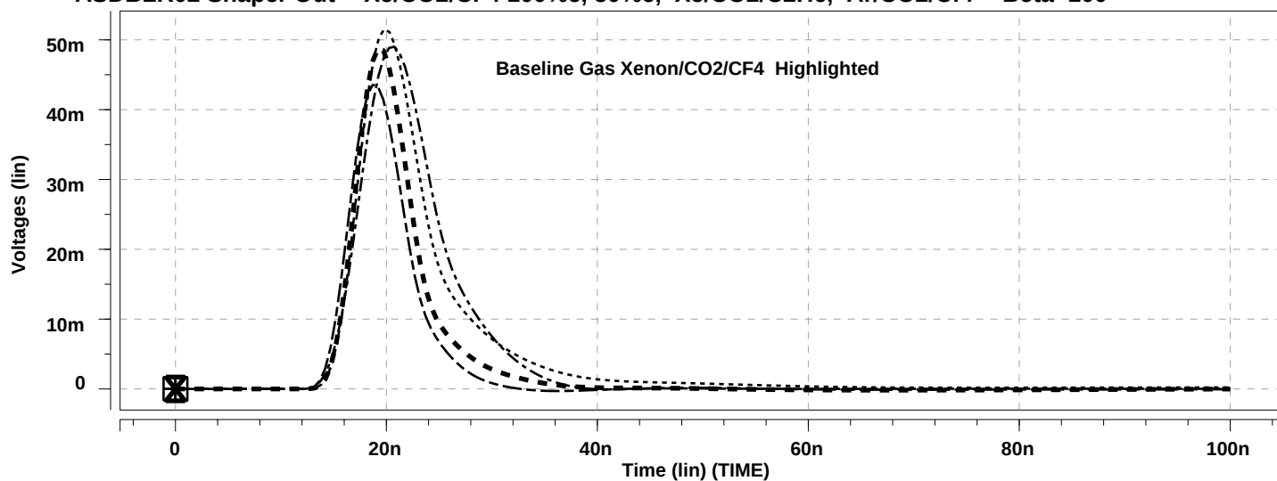
ASDBLR02 Disc Input -- Xe/CO2/CF4 100%e, 50%e, Xe/CO2/C2H6, Ar/CO2/Cf4 -- Beta=100
