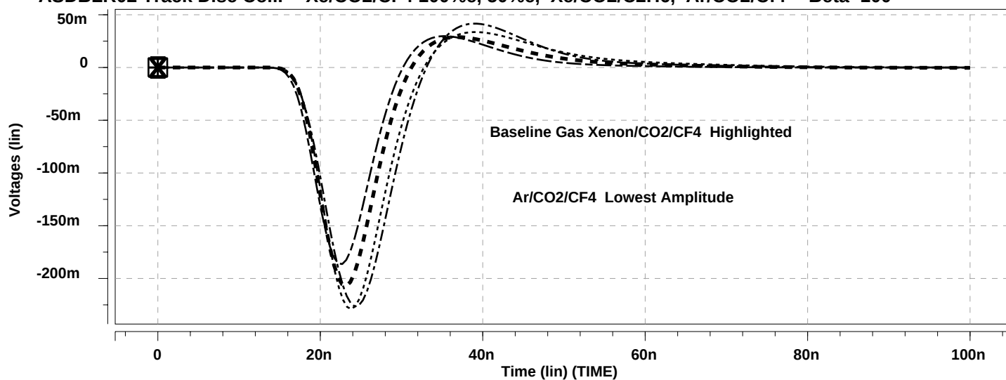
ASDBLR02 Track Disc Coll. -- Xe/CO2/CF4 100%e, 50%e, Xe/CO2/C2H6, Ar/CO2/Cf4 -- Beta=100
