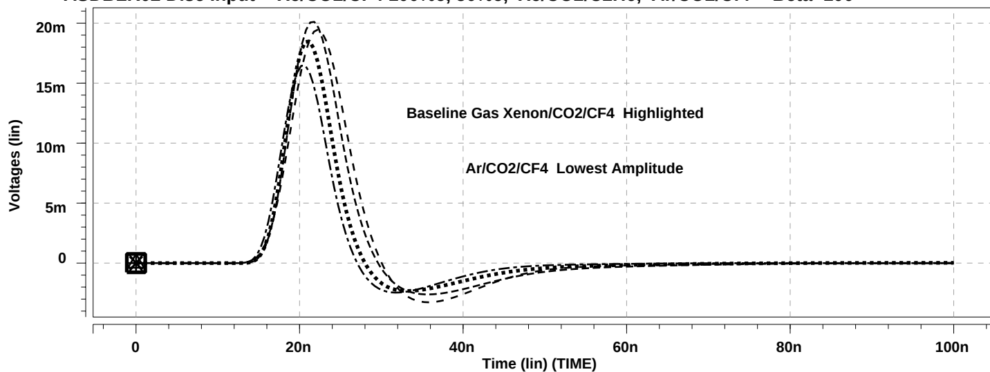
ASDBLR02 Track Disc Coll. -- Xe/CO2/CF4 100%e, 50%e, Xe/CO2/C2H6, Ar/CO2/Cf4 -- Beta=100
