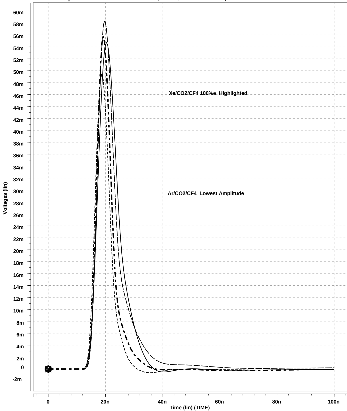
ASDBLR02 Shaper Out -- Xe/CO2/CF4 100%e, 50%e, Xe/CO2/C2H6, Ar/CO2/Cf4 -- Beta=250
