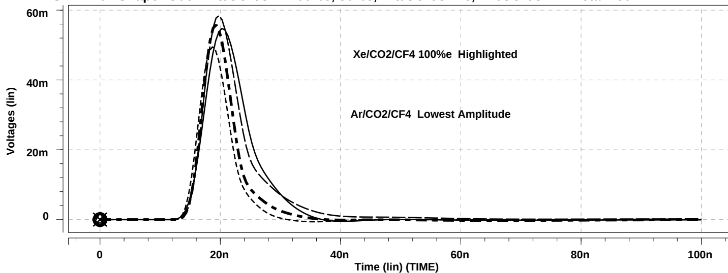
ASDBLR02 Disc Input -- Xe/CO2/CF4 100%e, 50%e, Xe/CO2/C2H6, Ar/CO2/Cf4 -- Beta=250
