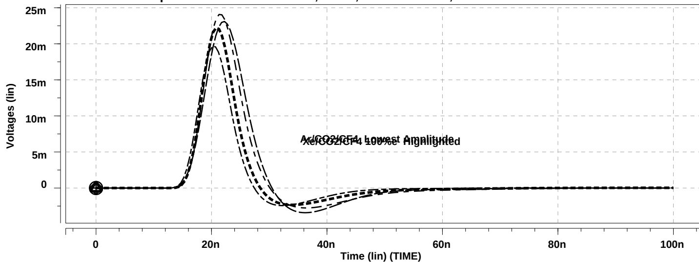
ASDBLR02 Track Disc Coll. -- Xe/CO2/CF4 100%e, 50%e, Xe/CO2/C2H6, Ar/CO2/Cf4 -- Beta=250
