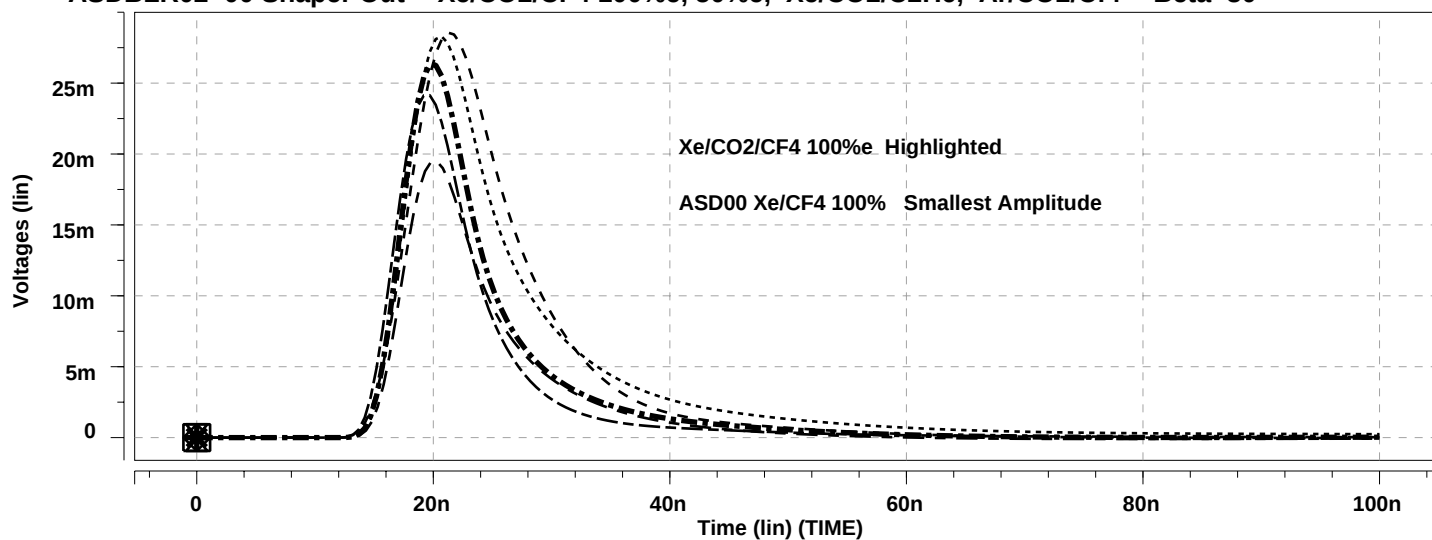
ASDBLR02+00 Disc Input -- Xe/CO2/CF4 100%e, 50%e, Xe/CO2/C2H6, Ar/CO2/Cf4 -- Beta=30
