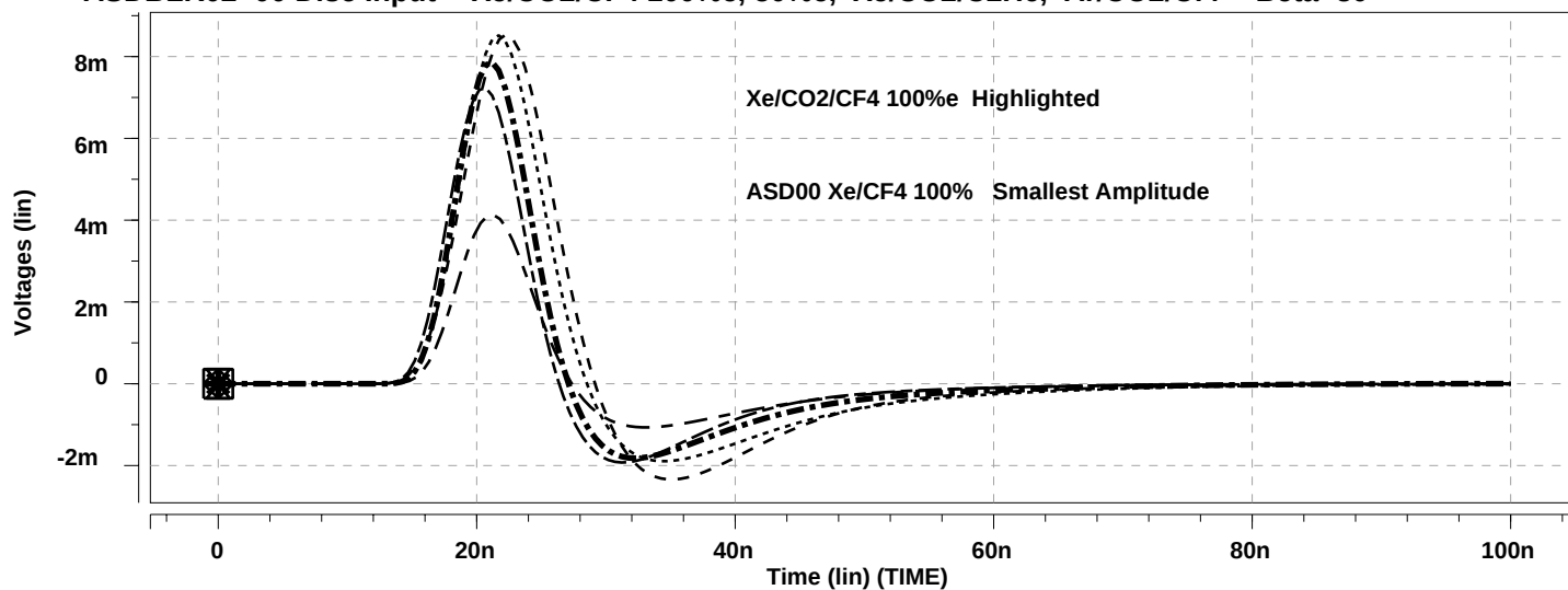
ASDBLR02+00 Track Disc Coll. -- Xe/CO2/CF4 100%e, 50%e, Xe/CO2/C2H6, Ar/CO2/Cf4 -- Beta=30
