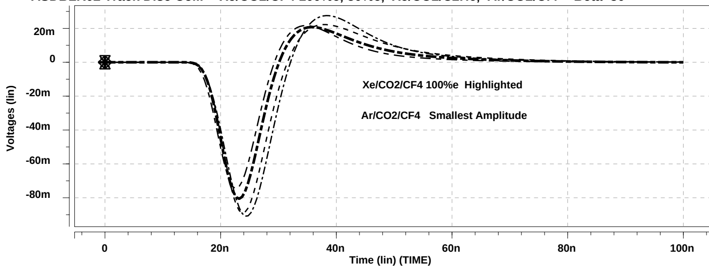
ASDBLR02 Track Disc Coll. -- Xe/CO2/CF4 100%e, 50%e, Xe/CO2/C2H6, Ar/CO2/Cf4 -- Beta=30
